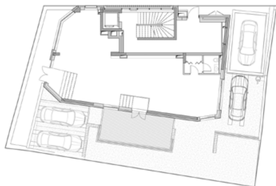
Разпределение етаж 1
