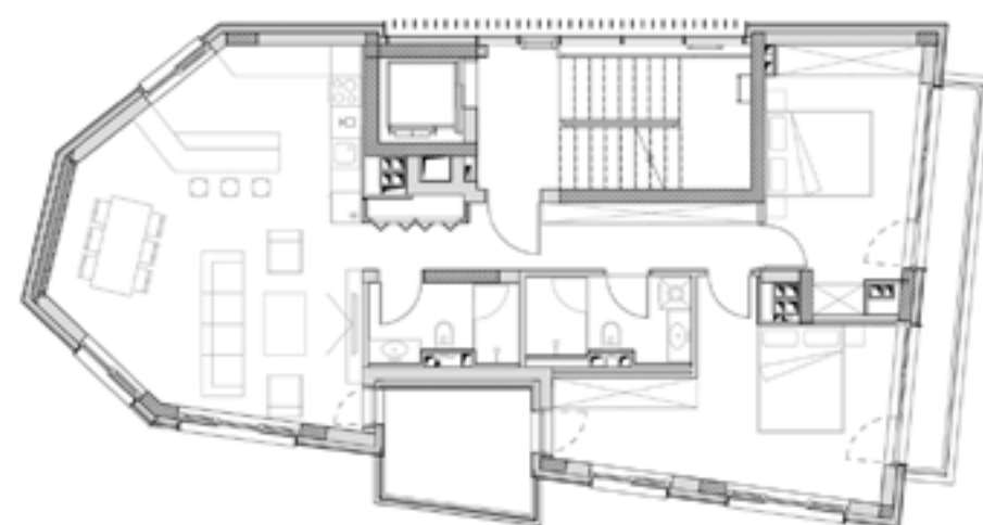
Разпределение етаж 5
